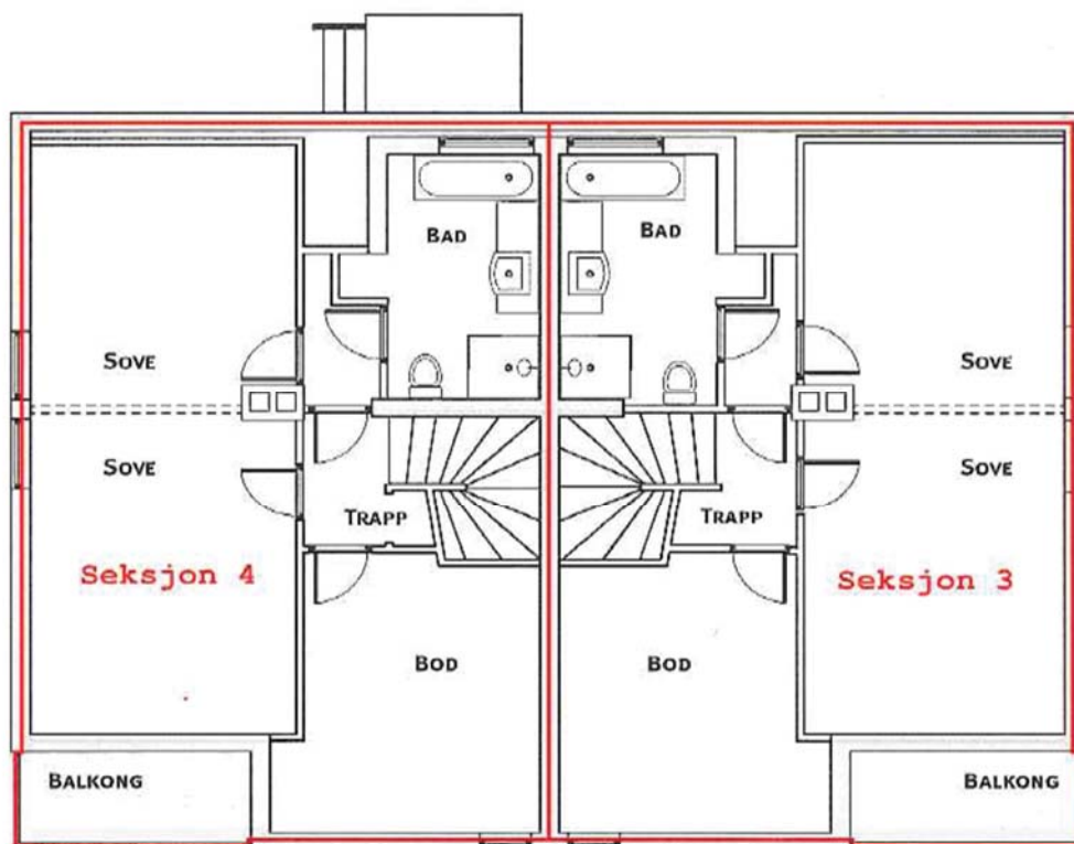
Loft
