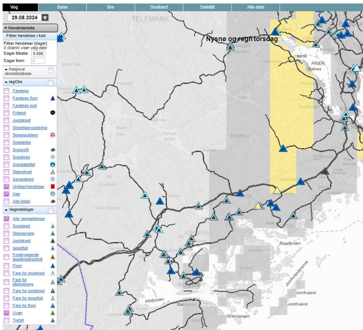
Figur 4-12: Xgeo oversikt historiske uværsmeldinger siste 5000 dager (xgeo.no) [16].
