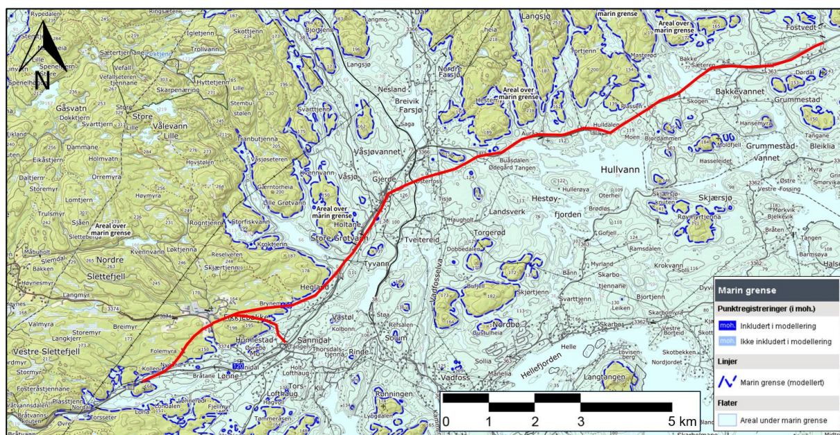
Figur 4-3 Utklipp av NGUs kvartærgeologiske kart påført arealer under marin grense. Prosjektert E18 er påført som rød linje. (kilde: [8].
