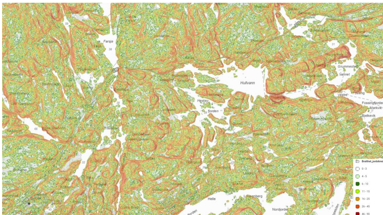
Figur 4-5 Bratthetskart for jordskred langs prosjektert E18 [10]
