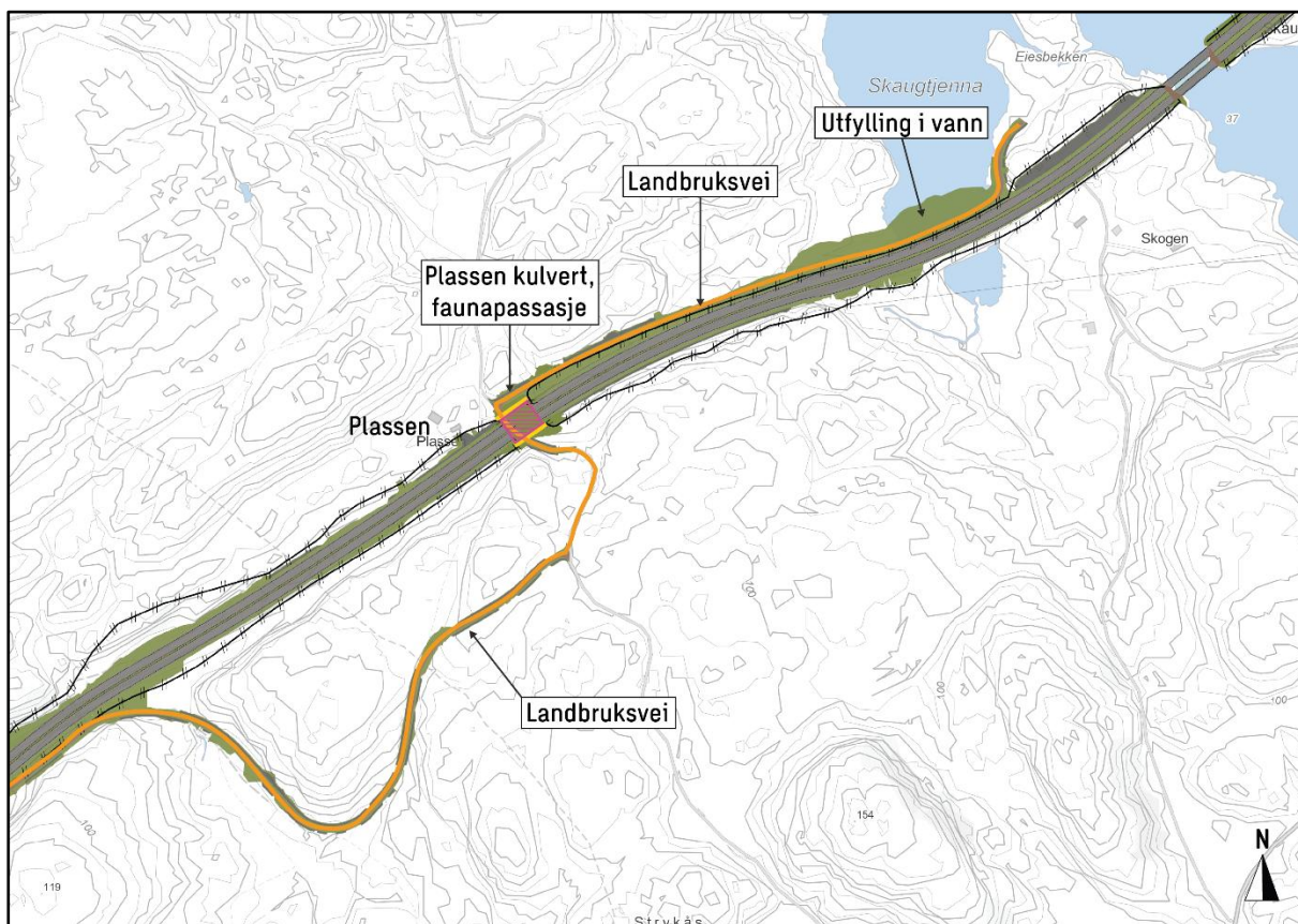
Figur 3-41: Tiltak ved Plassen og Skaugtjenna (Kilde: Sweco)
