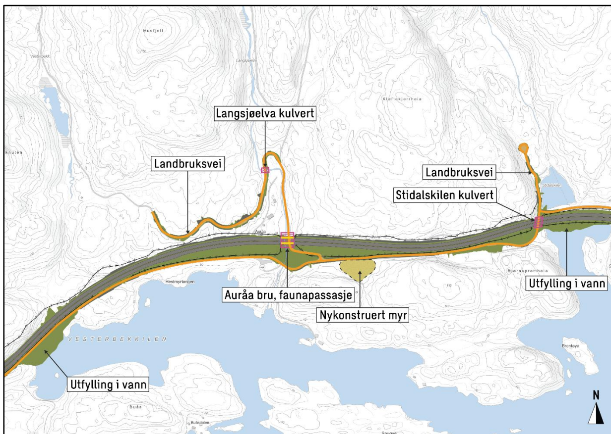
Figur 3-33: Planlagte tiltak langs Hullvann. (Kilde: Sweco)
