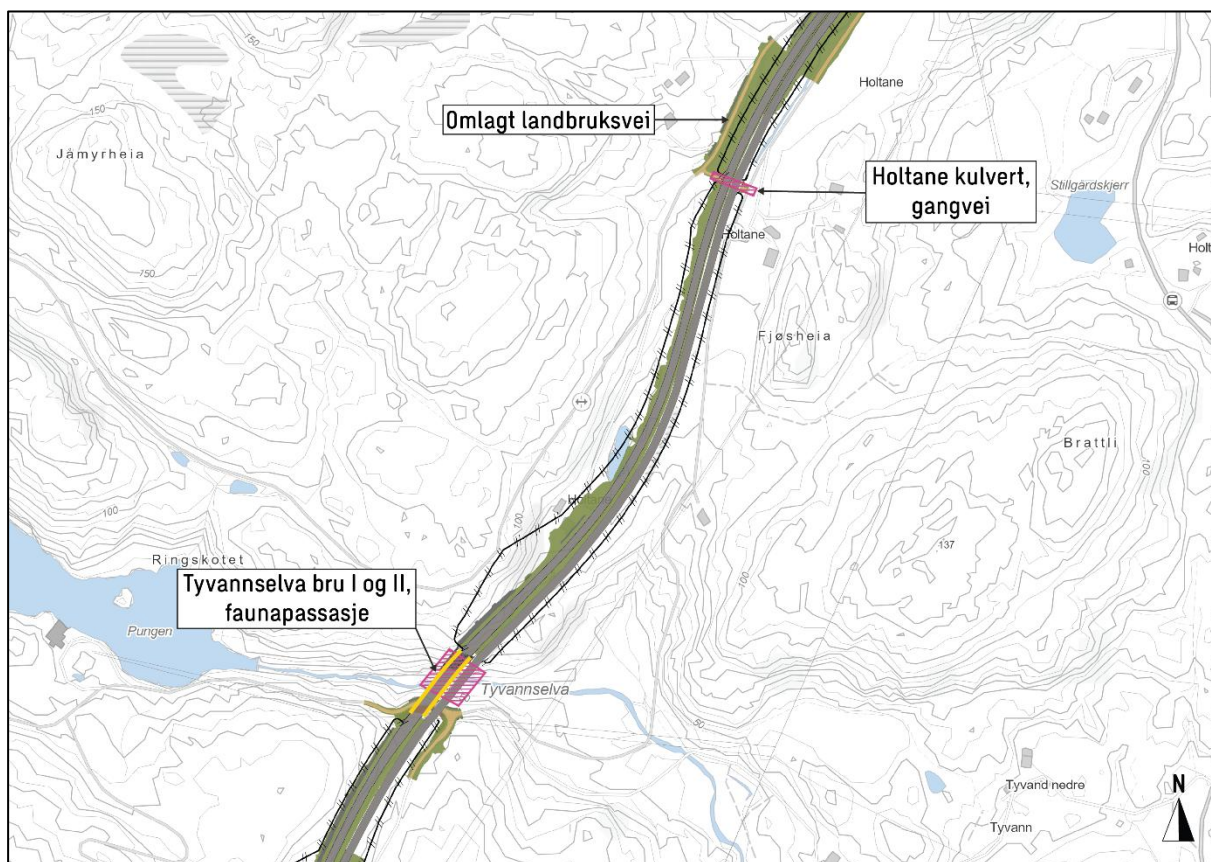
Figur 3-22: Tiltak ved Tyvannselva og Holtane. (Kilde: Sweco)
